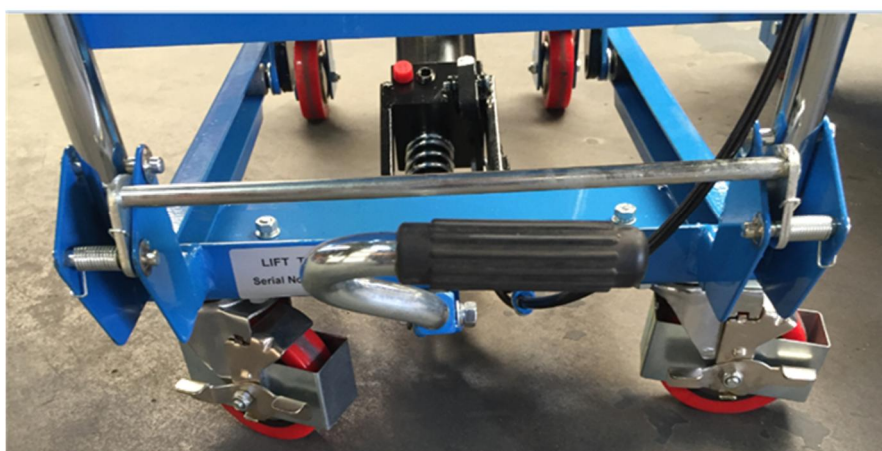
Pedale à pied de montée, 2 roues pivotantes a Freins papillons
